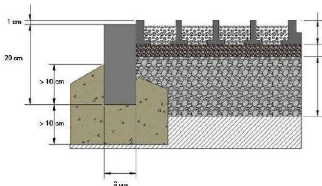
Boordsteen type 1 op niveau Afgewerkt hoogte is 1 cm boven de roosters. *Maten in de tekeningen zijn volgens de Franse normen.
