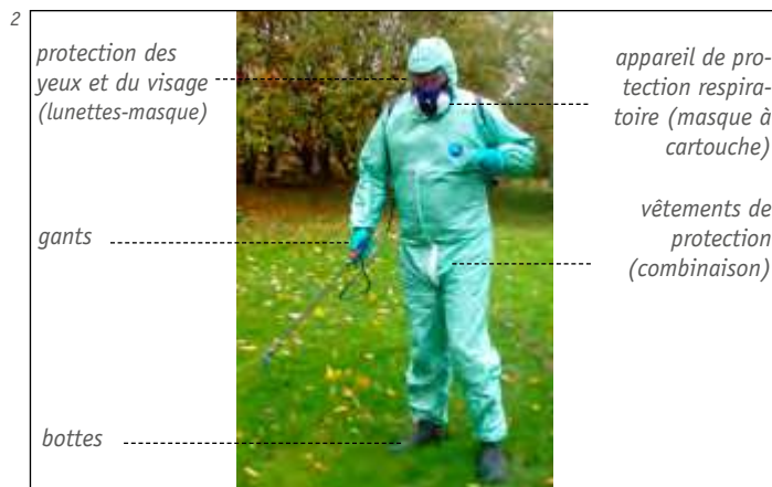
2 - Agent applicateur portant les équipements de protection individuelle (EPI) obligatoires. © P&C - Maxime GUERIN 2014
