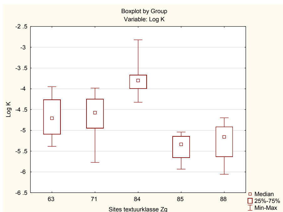
Figuur 3-16: Box plot die de gemiddelde Log K met de spreiding aanduidt voor de verschillende sites binnen textuurklasse Zg.
