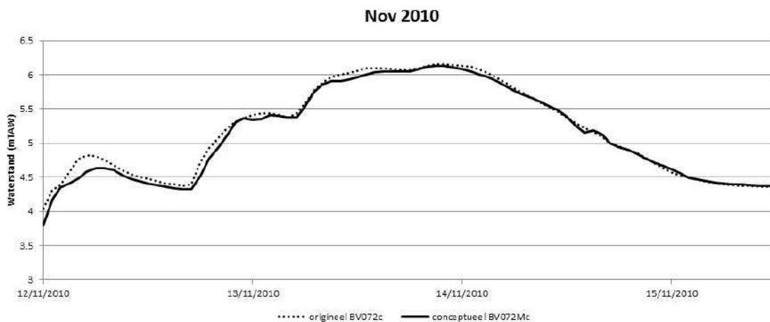
Figuur 4-19: Overzicht van de waterpeilen in de Benedenvliet ter hoogte van de Cleydaellaan te Aartselaar in het volledig hydrodynamisch en het conceptueel waterloopmodel voor een periode in november 2010 met een terugkeerperiode van 25 jaar
