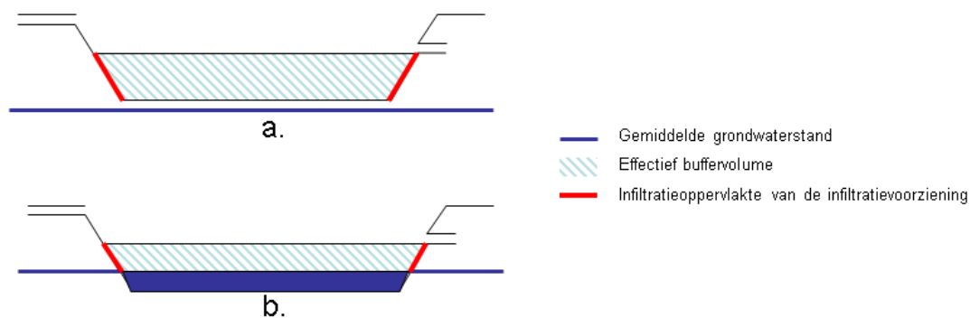
Figuur a: Aanleg van een infiltratiebekken boven de grondwatertafel
